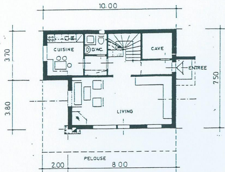
REZ-DE-CHAUSSÉE
