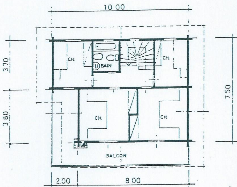
ÉTAGE
